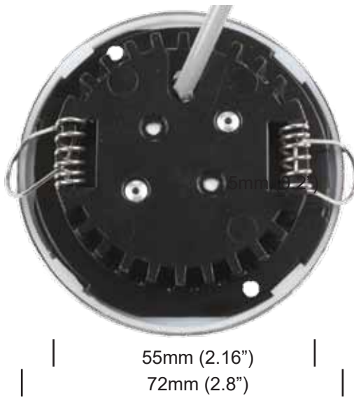
ROUND BEZEL
